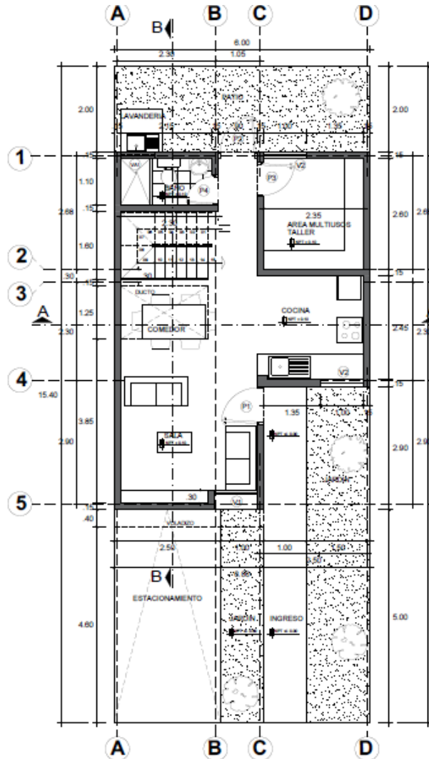
PLANO PLANTA NIVEL o 1
