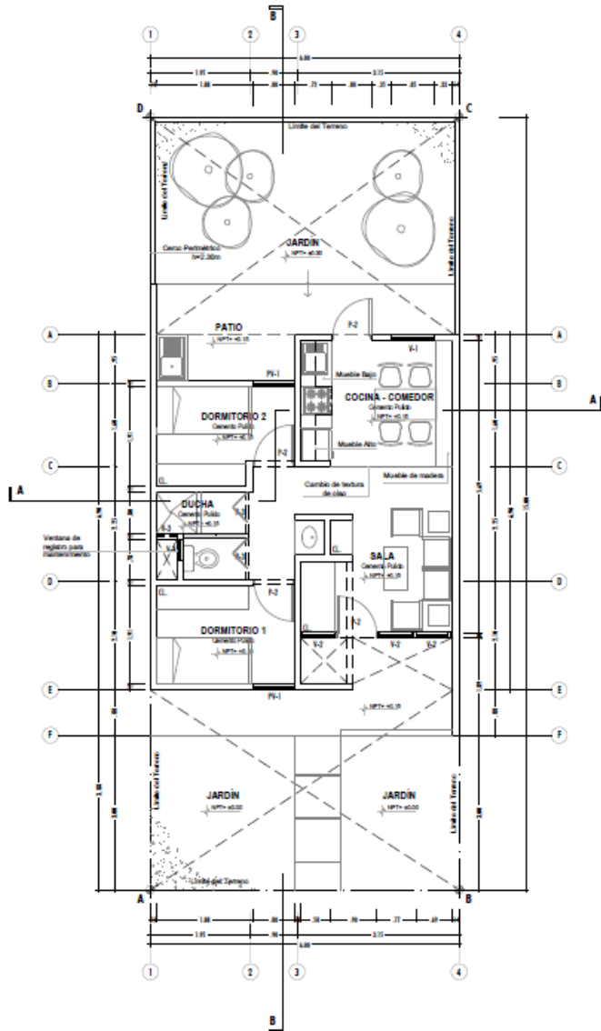
MÓDULO BÁSICO 38.29 M2
