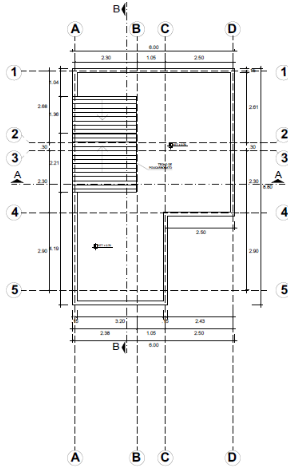
PLANO DE TECHO
