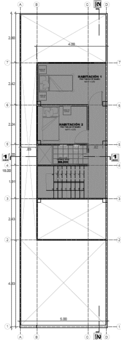
SEGUNDO NIVEL
