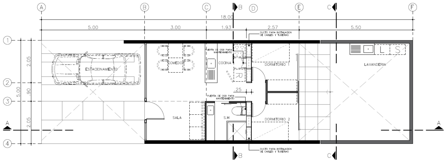
MÓDULO BÁSICO 36.50 M2
