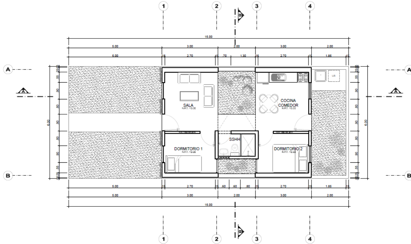
MÓDULO BÁSICO 38.40 M2
