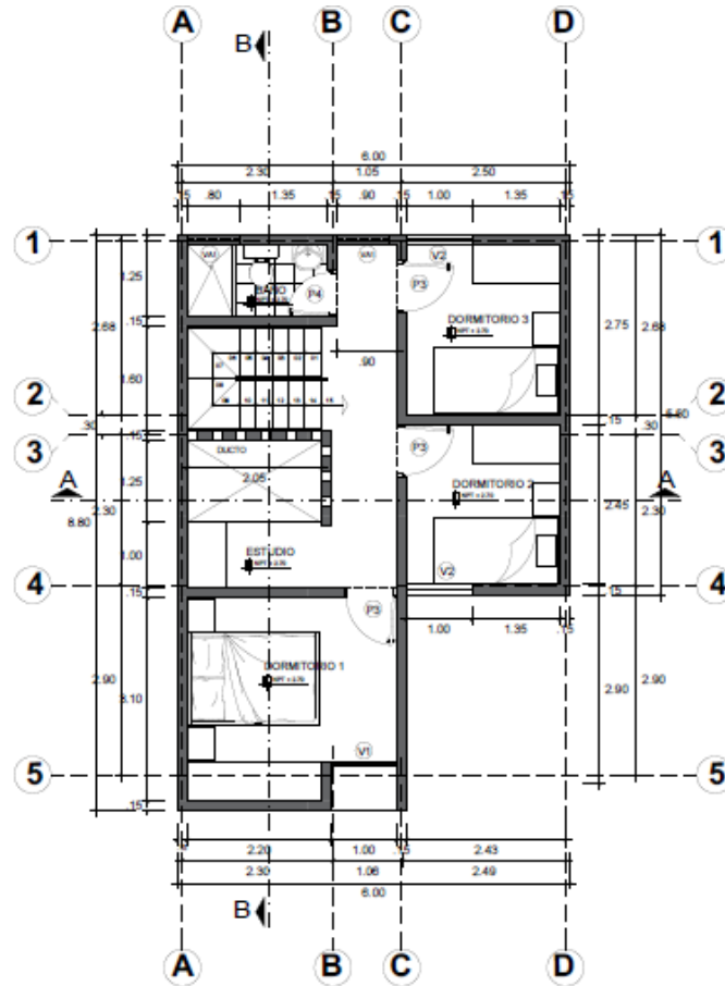
PLANO PLANTA NIVEL o 2
