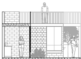
CORTE B-B
