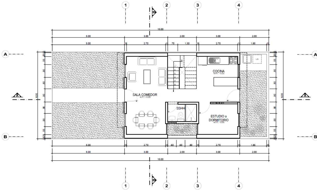
MÓDULO CON CRECIMIENTO PROGRESIVO 81.05 M2
