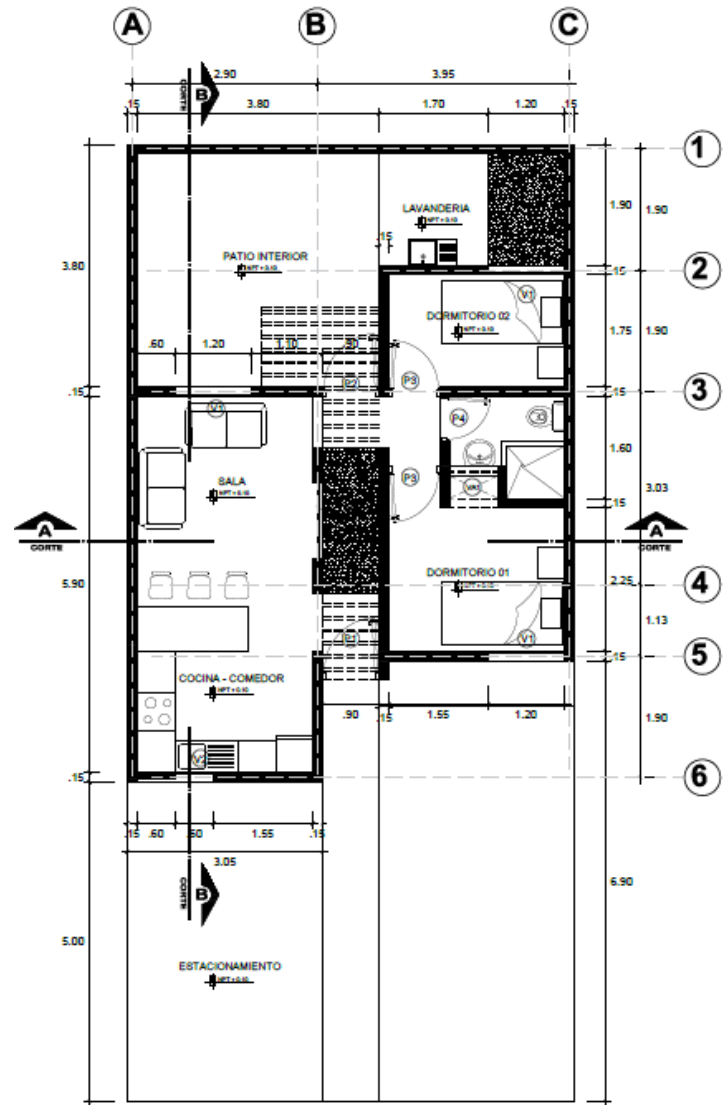
MÓDULO BÁSICO 38.00 M2
