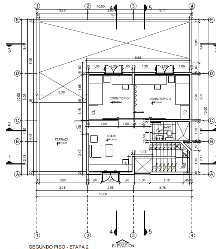
SEGUNDO PISO - ETAPA 2
