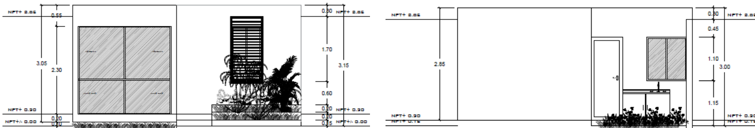
ELEVACIÓN POSTERIOR
