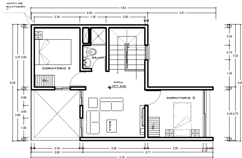
PLANTA SEGUNDO NIVEL
