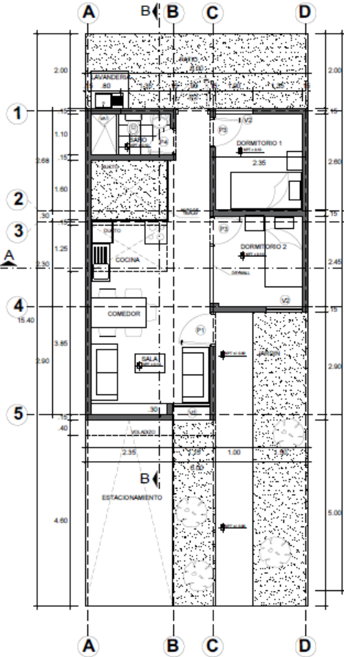
PLANO PLANTA NIVEL 0 1
